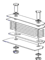
ENSAMBLE PLACAS GUIA
